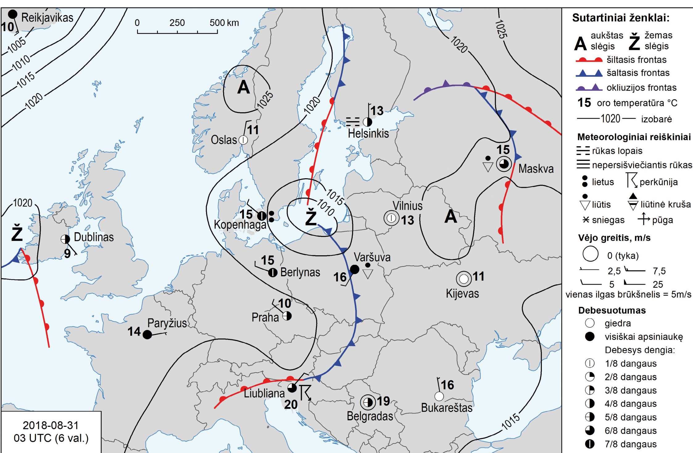
Europos sinoptinis žemėlapis
