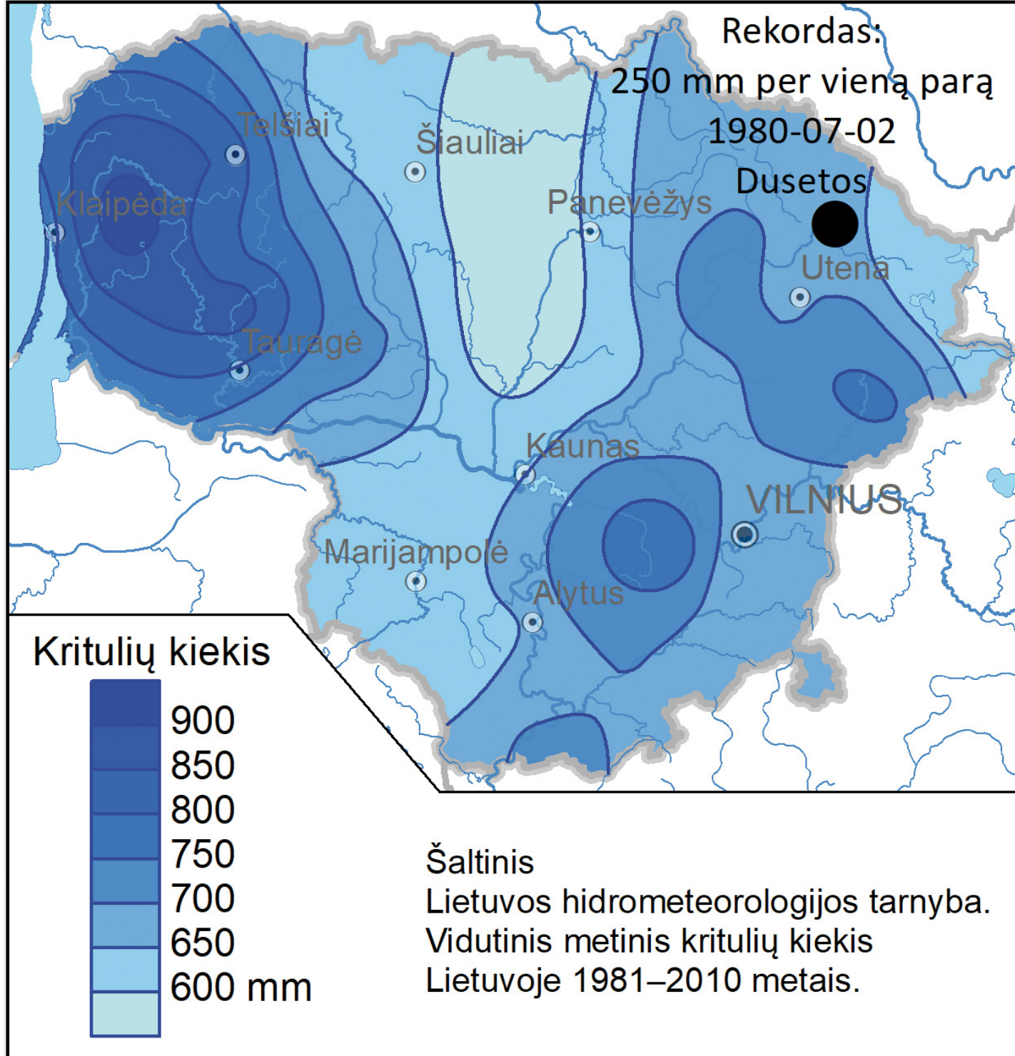
Vidutinis metų kritulių kiekis
