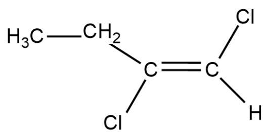
1,2-dichlorobut-1-en
